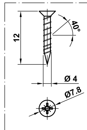
Tirafondos POZ Ø4x12 Screw POZ Ø4x12
