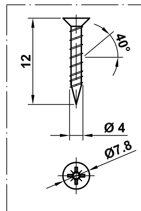
Tirafondos POZ Ø4x12 Screw POZ Ø4x12
